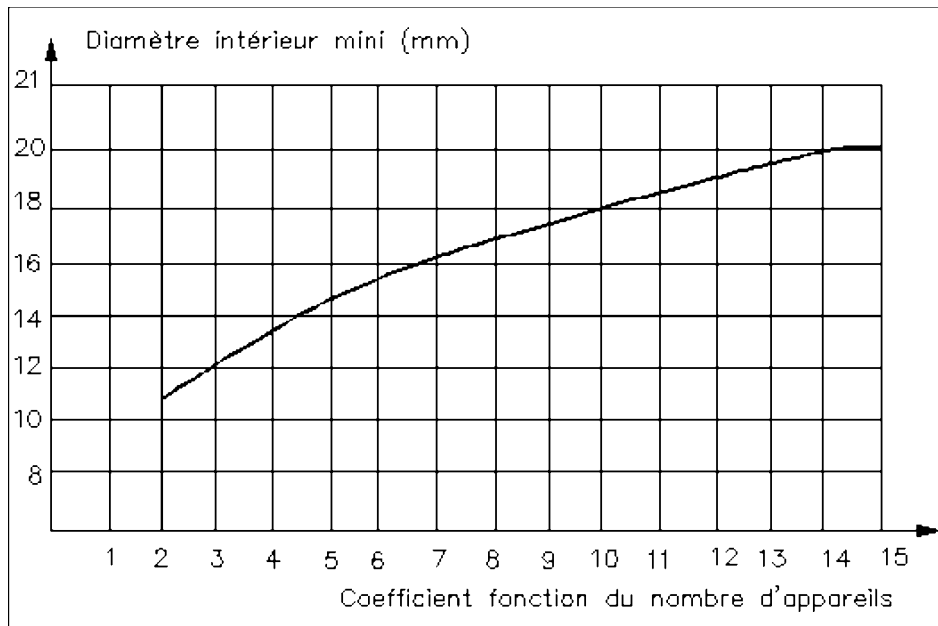
Diamètre intérieur minimal d'alimentation en fonction du nombre d'appareils Parties individuelles
