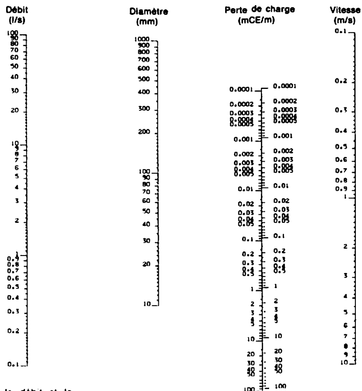
Abaque pour le calcul des conduites d'eau chaude
