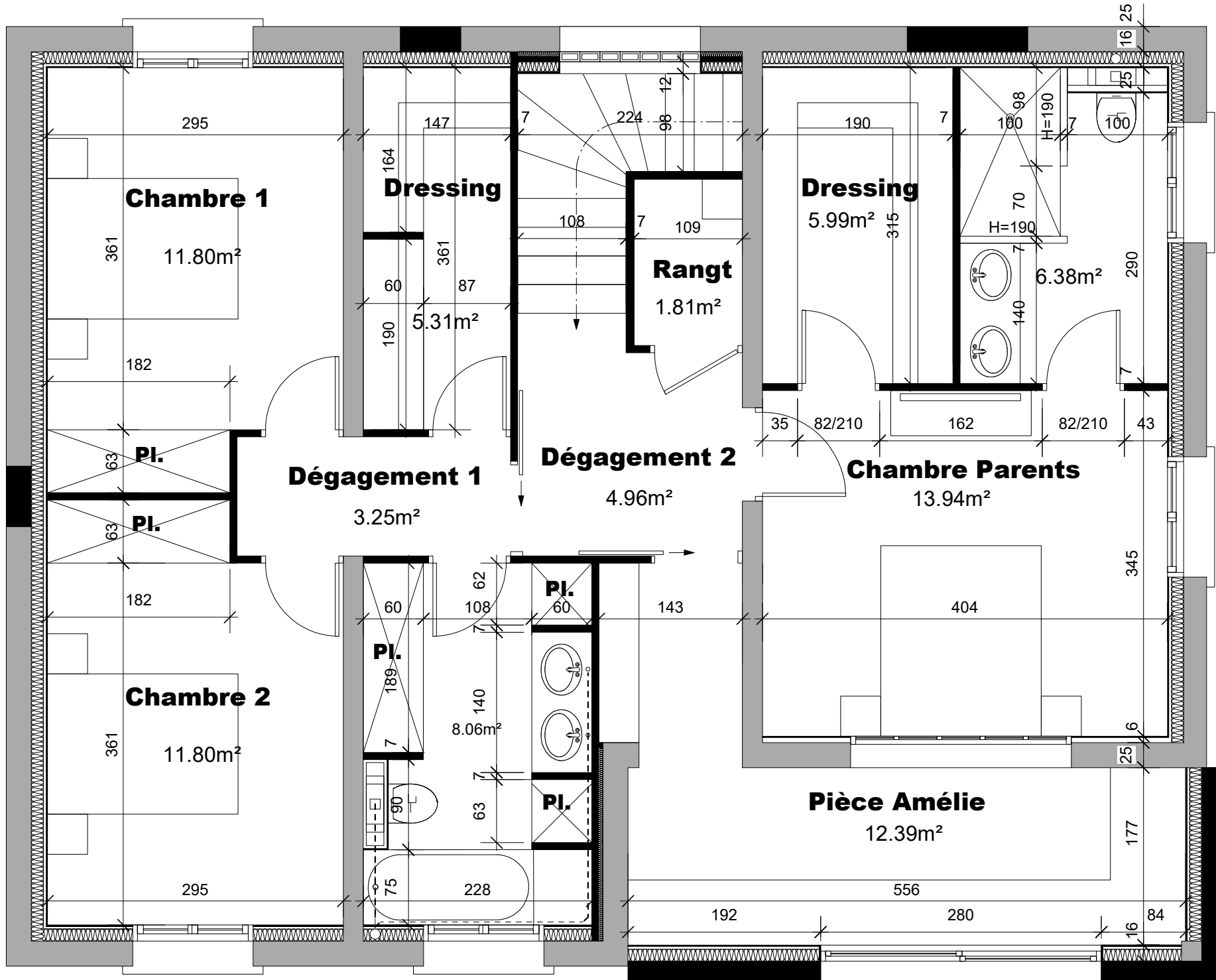
PLAN ETAGE - échelle 1/50
