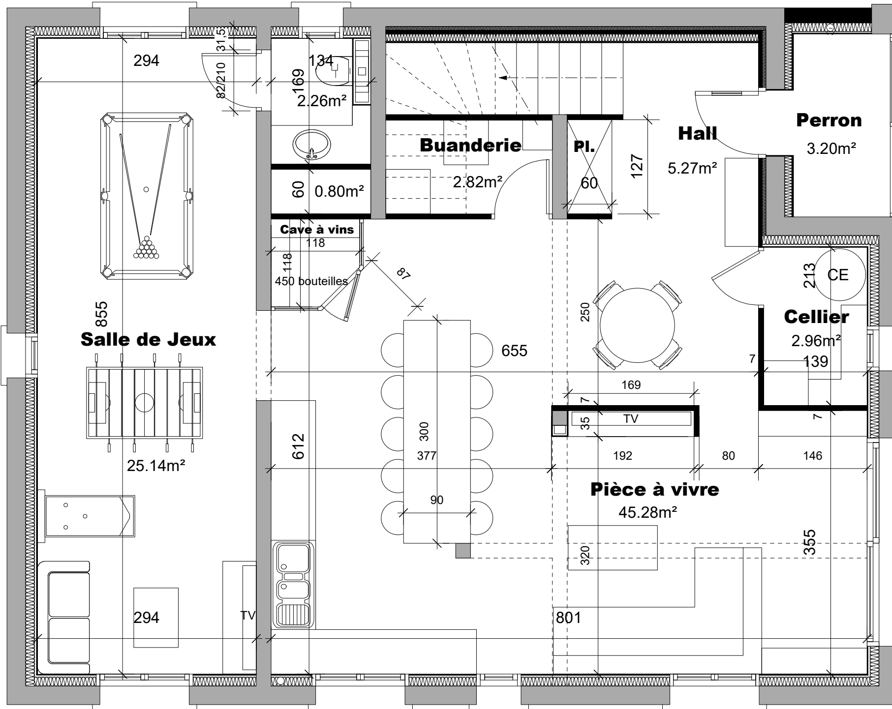
PLAN REZ DE CHAUSSEE - échelle 1/50
