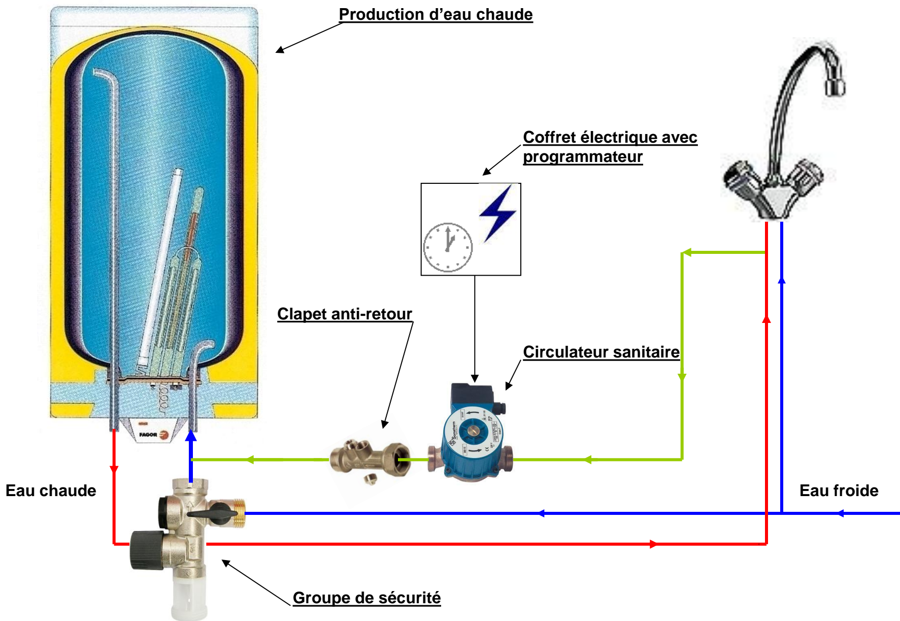
Schéma de principe d'un bouclage sanitaire
