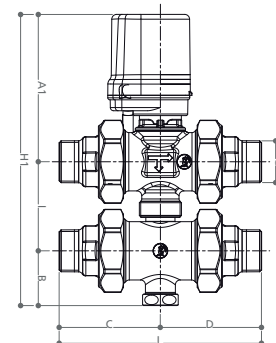
Encombrement avec tête électrothermique R473 ou R478
