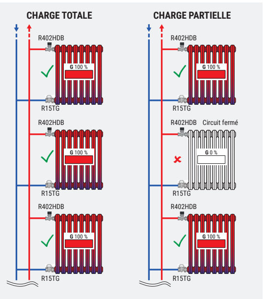
Système de colonne montante avec robinets série DB, avec équilibrage dynamique
